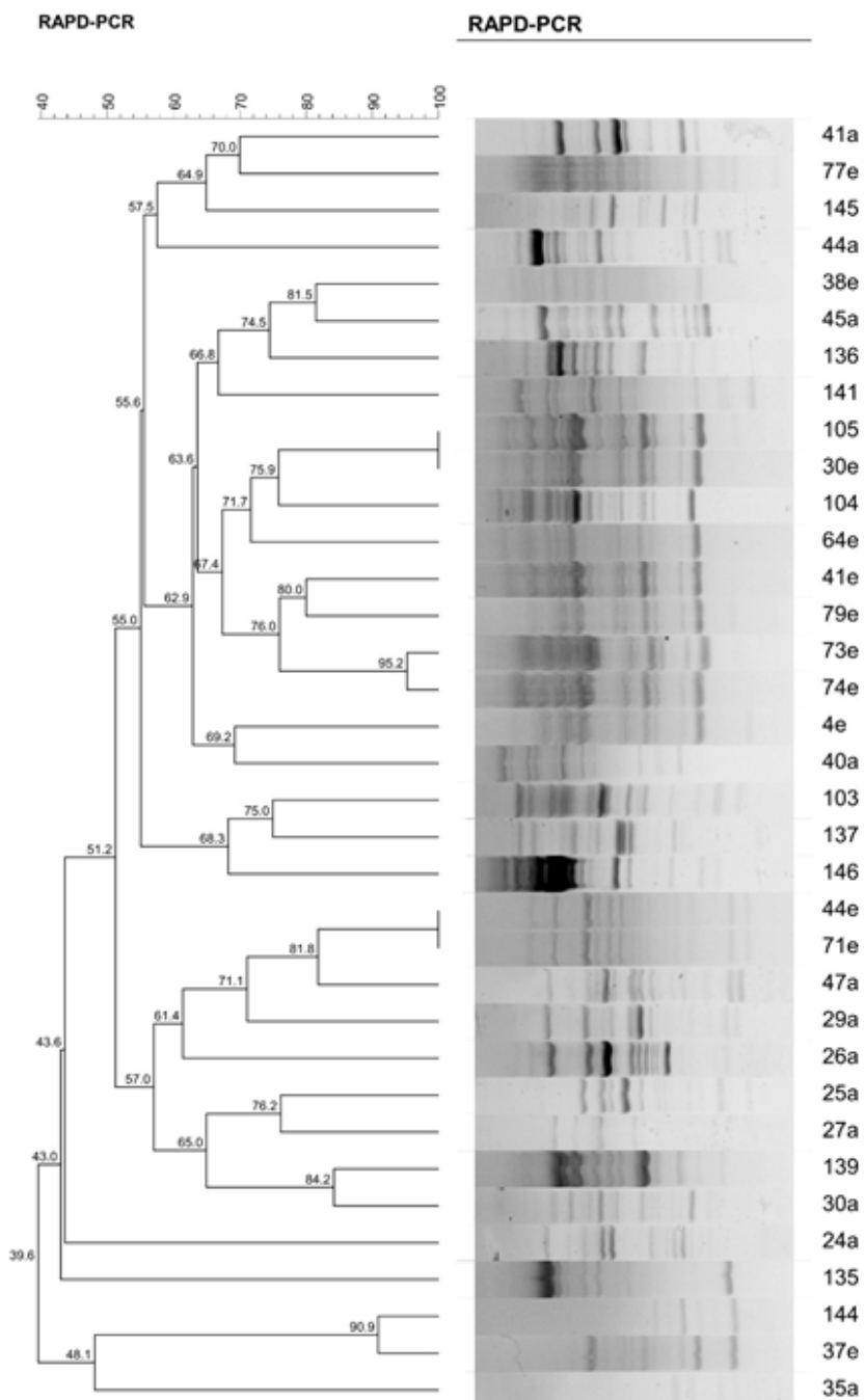
شکل ۳: دندروگرام ارتباط ژنتیکی بین سرگروپ‌های O25 باکتری/شریشیالکی براساس نشانگر RAPD-PCR
