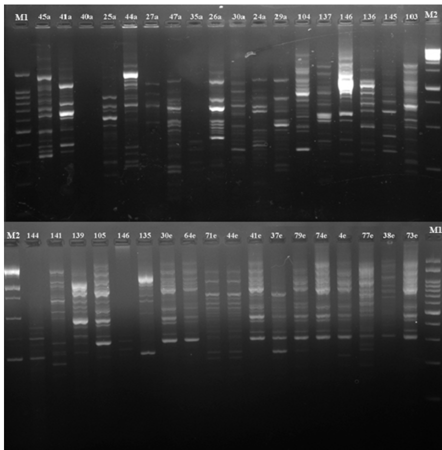
شکل ۲: باندهای حاصل از آنالیز RAPD-PCR مربوط به سرگروپ‌های O25 باکتری اشریشیکلی (ستون M1= مارکر ۱۰۰ جفت بازی DNA؛ ستون M2= مارکر ۱ کیلوبازی DNA)
